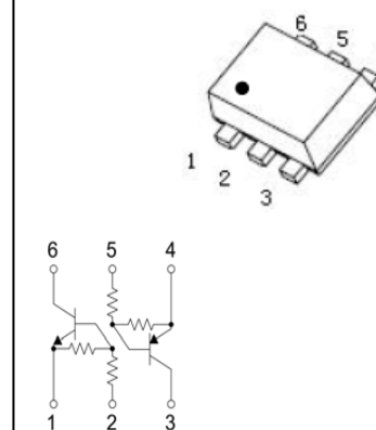
SOT-563
